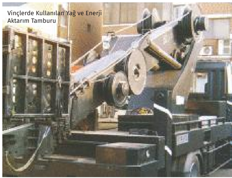
Vinçlerde Kullanılan Yağ ve Enerji Aktarım Tamburu
